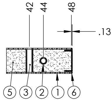
SECTION A-A SCALE 1 : 8
