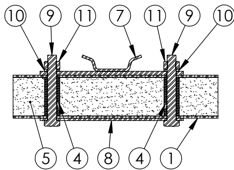
SECTION B-B SCALE 1 : 8
